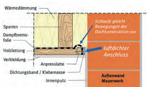
Beispiel für einen dauerhaft dichten Wandanschluss einer Dampfbremsfolie an die Giebelwand im Dachgeschoss bei bestehendem Innenputz
